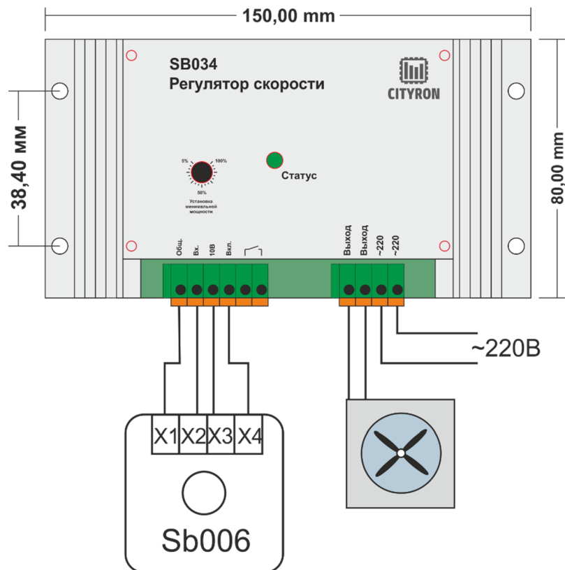
Схема 3 Управление внешним сигналом 0-10V от любого контроллера с выходом 0-10V
