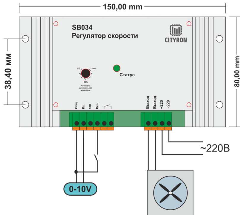
Схема 3 Управление внешним сигналом 0-10V от любого контроллера с выходом 0-10V
